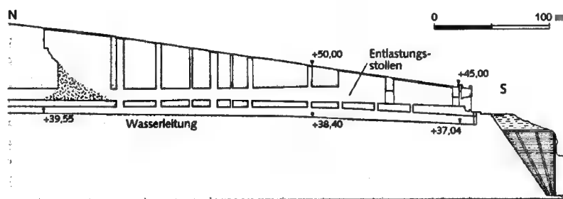
Abb. 1: Syrakusai. Doppelstollen der Ninfeo-Leitung, spätklass.; südl. Abschnitt (Schnitt).
